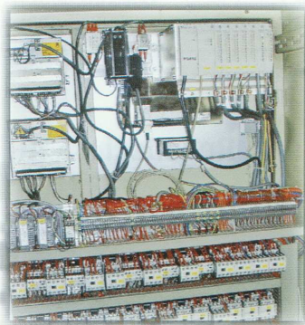
Moeller-Steuerung zur Energiemessung
